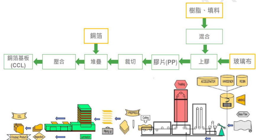
圖一、PCB 銅箔基板與膠片製程
